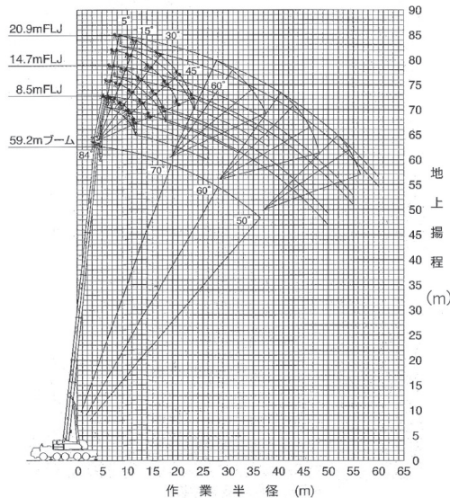
59.2mブーム+1.85m+フルオートラフingジブ
