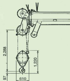
25 tフック 450kg
