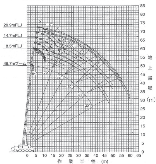
46.7mブーム+1.85m+フルオートラフingジブ
