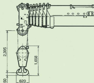
125 tフック 1,350kg
