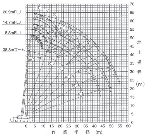
38.3mブーム+1.85m+フルオートラフィングジブ
