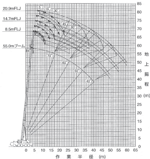
55.0mブーム+1.85m+フルオートラフingジブ
