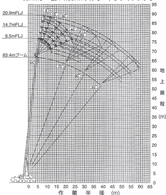
63.4mブーム+1.85m+フルオートラフingジブ
