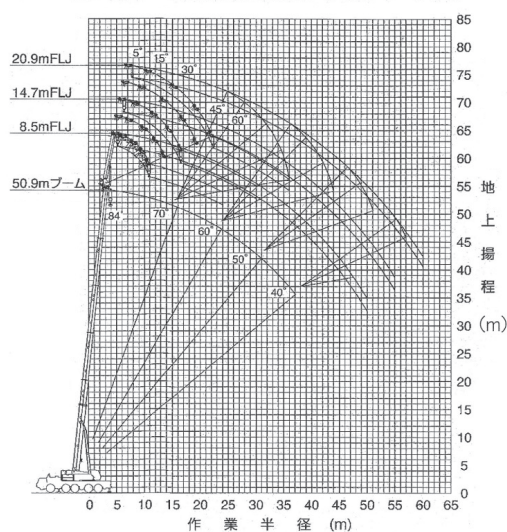
50.9mブーム+1.85m+フルオートラフingジブ
