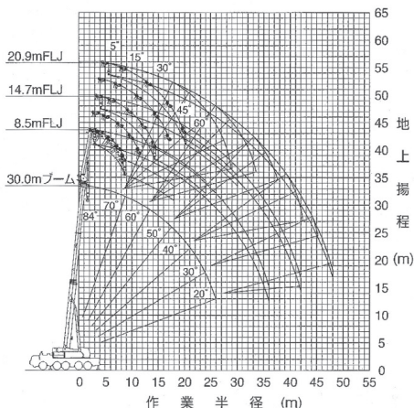
30.0mブーム+1.85m+フルオートラフィングジブ
