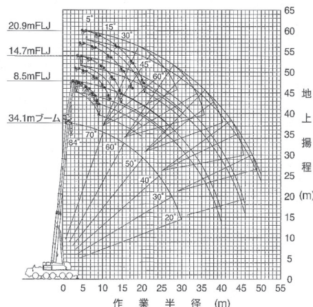
34.1mブーム+1.85m+フルオートラフィングジブ
